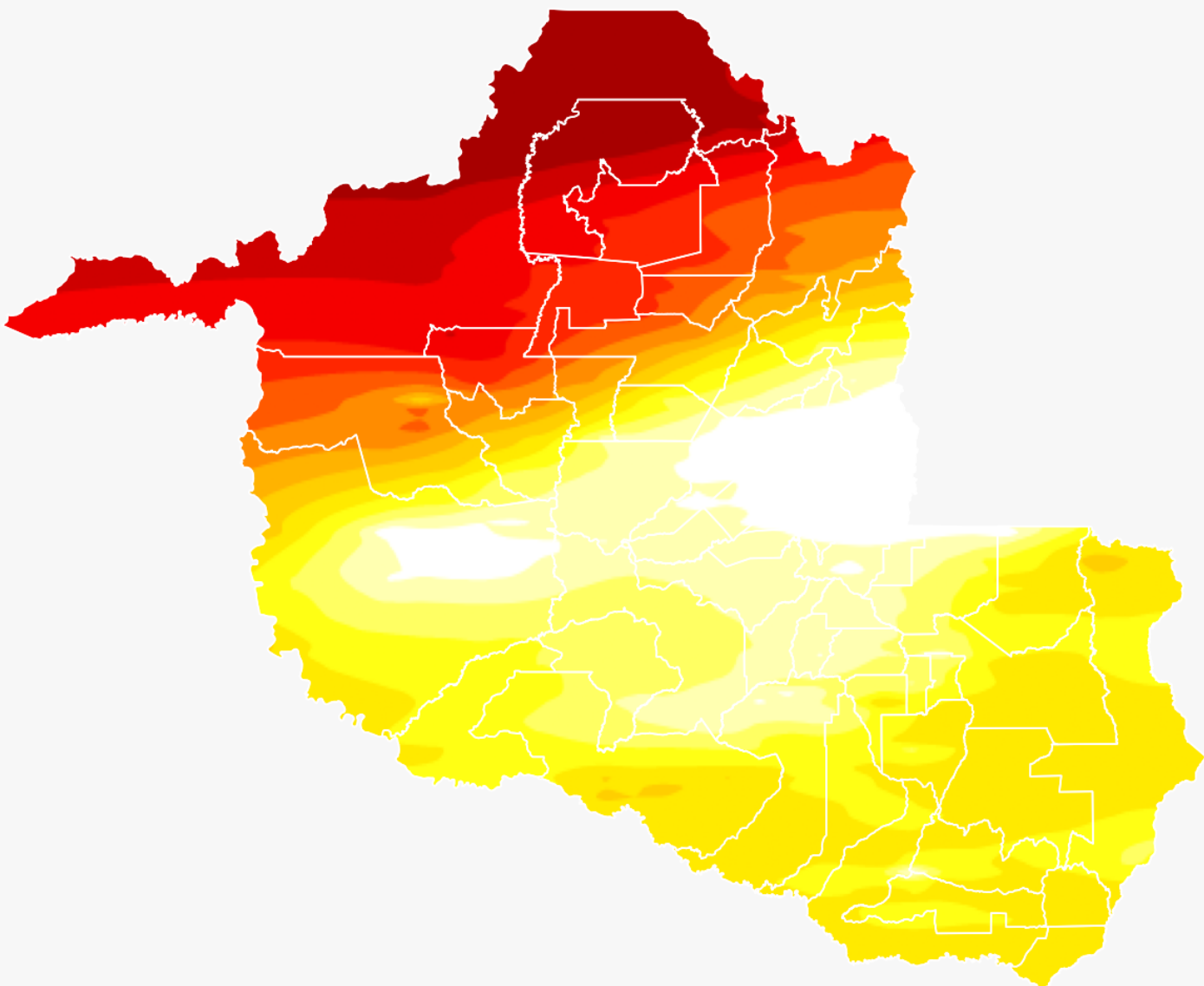
ENERGISA Rondônia Previsão de Anomalia de Temperatura Mínima 11 de Jun
