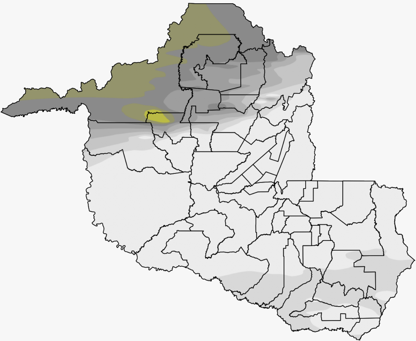
ENERGISA Rondônia Previsão de Onda de Calor de 7 de Jun até 13 de Jun
